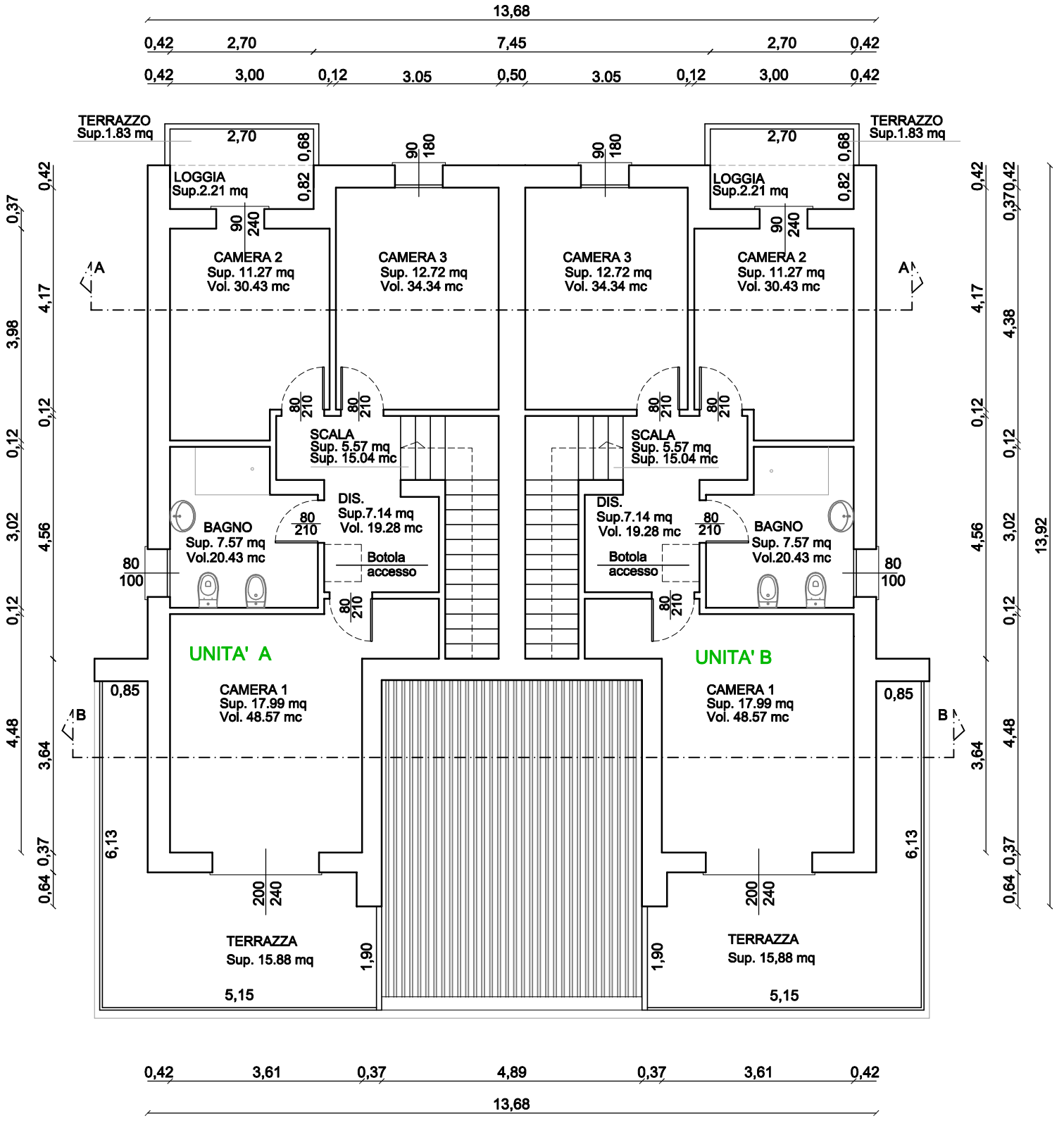
PIANTA PIANO PRIMO Scala 1:100
