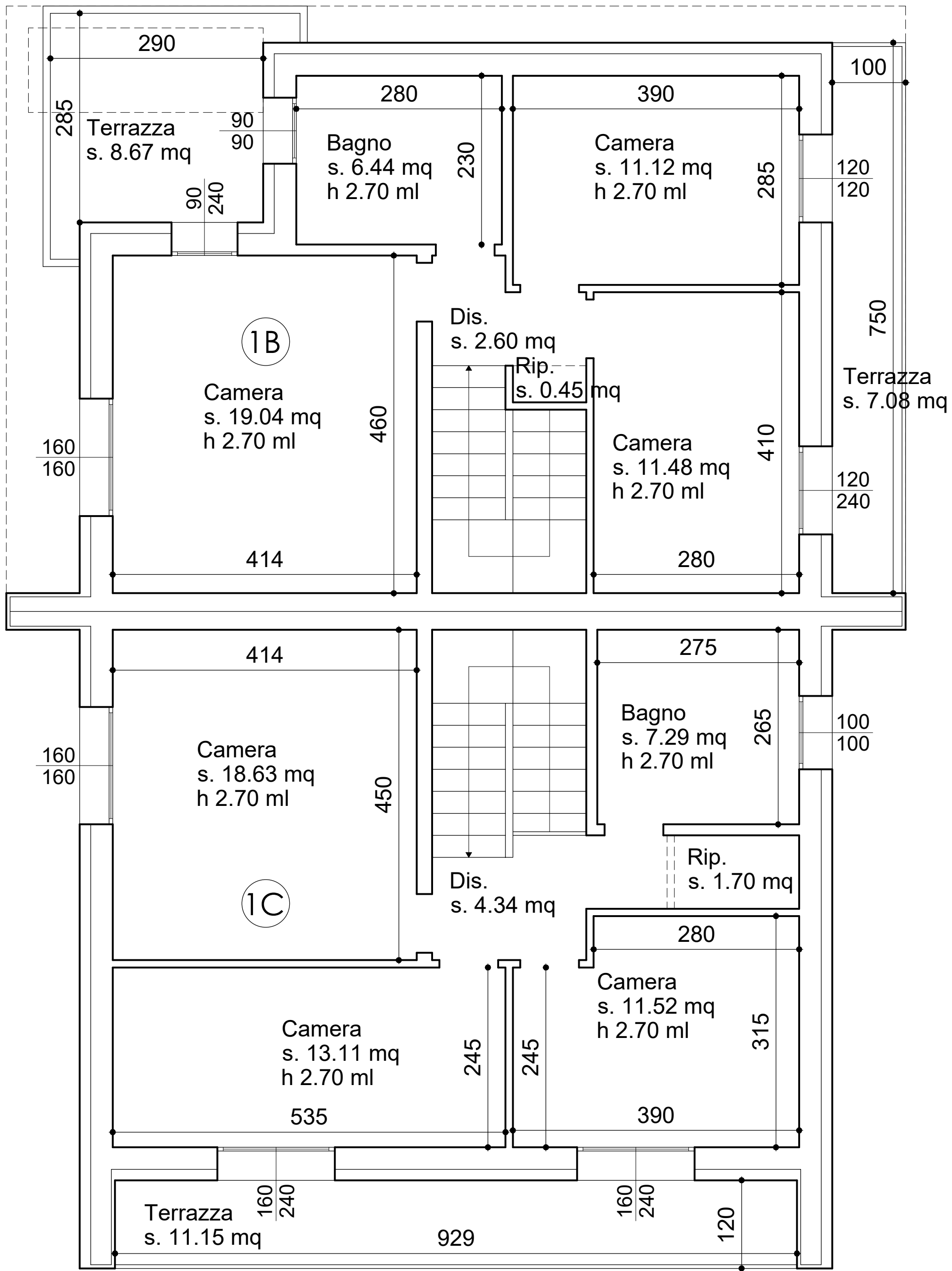
Pianta piano primo Scala 1:50
