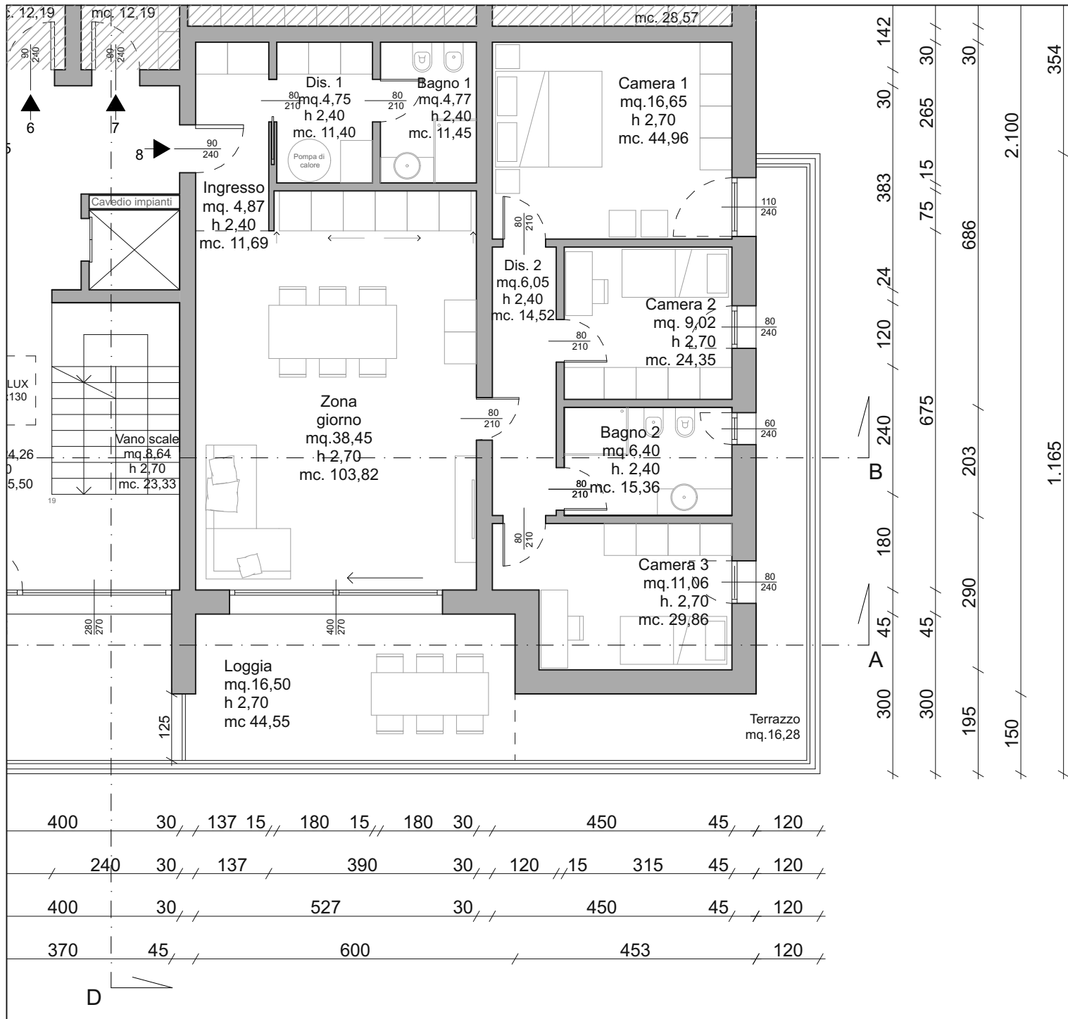
Pianta Appartamento 8 Secondo Piano scala 1:100 24_01_24
